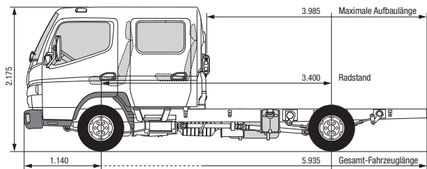
Doppelkabine: 3C13D, 3C15D
