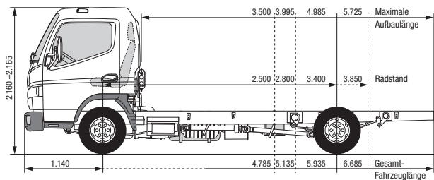
Seitenansicht Einzelkabine: 3C13, 3S13, 3C15, 3S15
